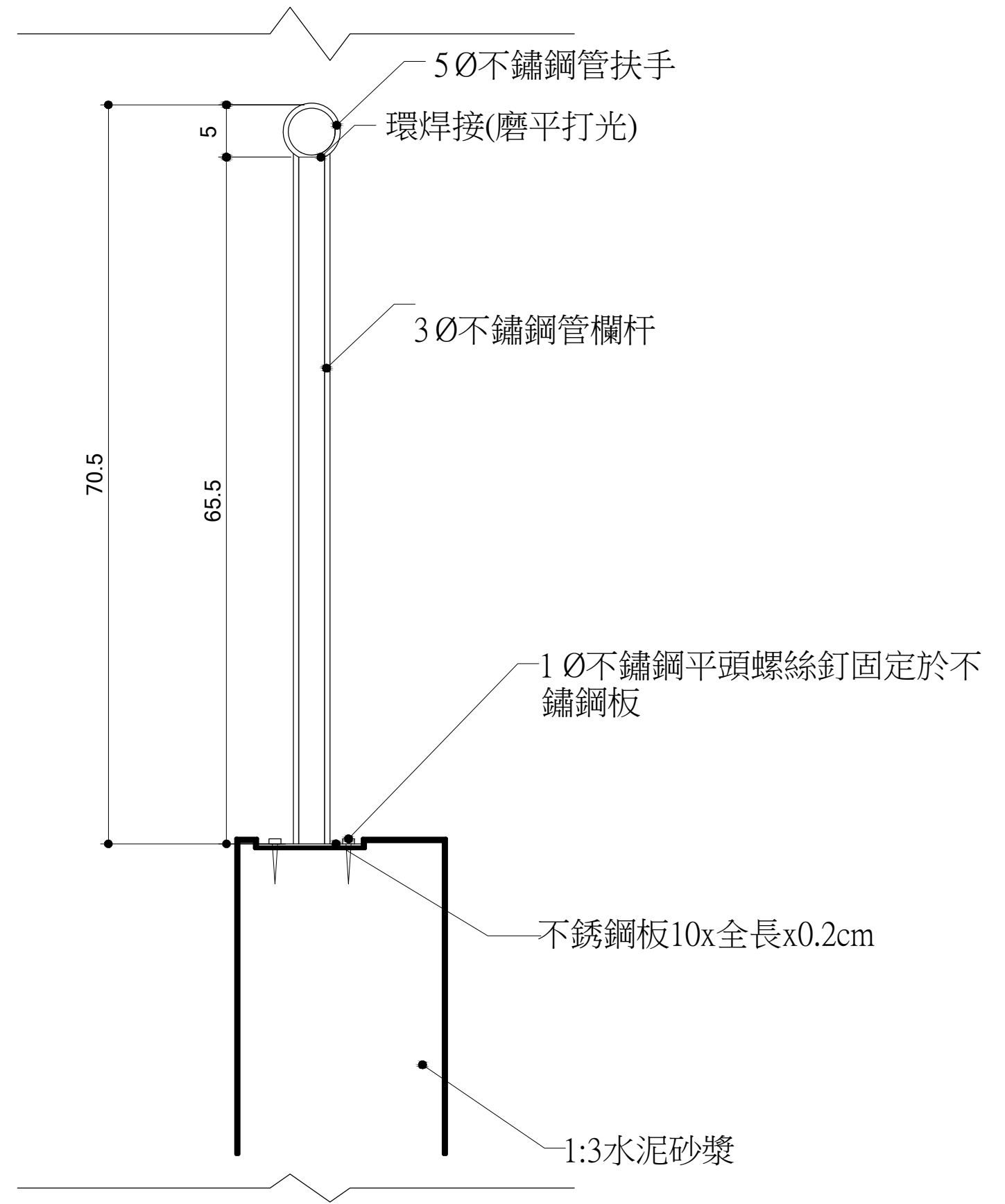
② 細部大樣改善詳圖S=1:5
