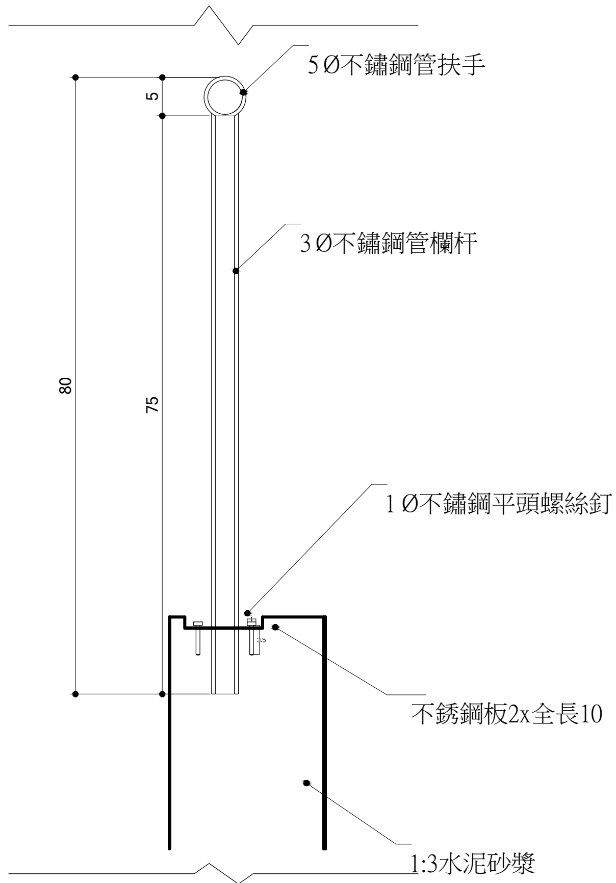
① 細部大樣詳圖S=1:5
