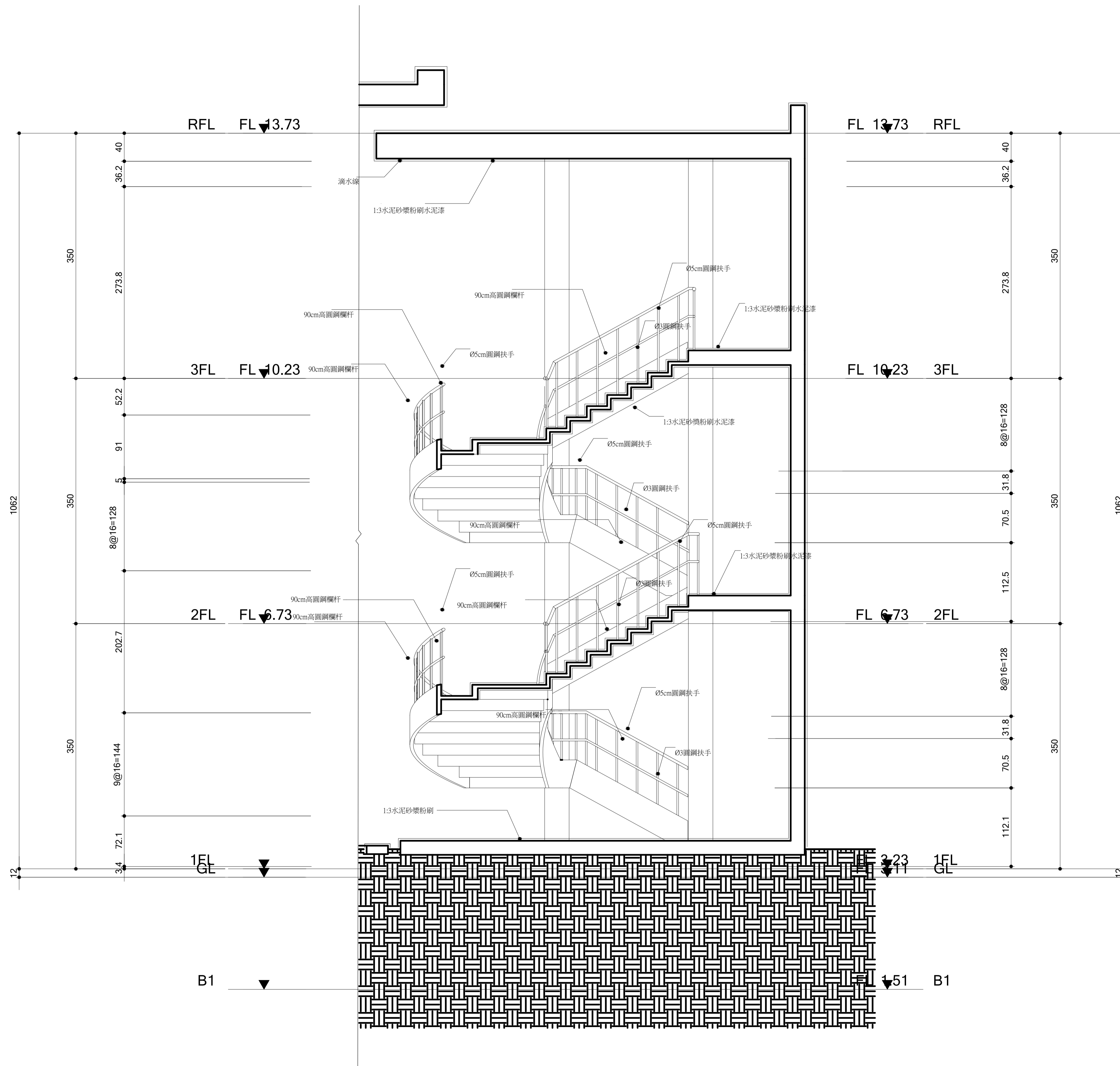
旋轉樓梯剖面詳圖 S=1:30
