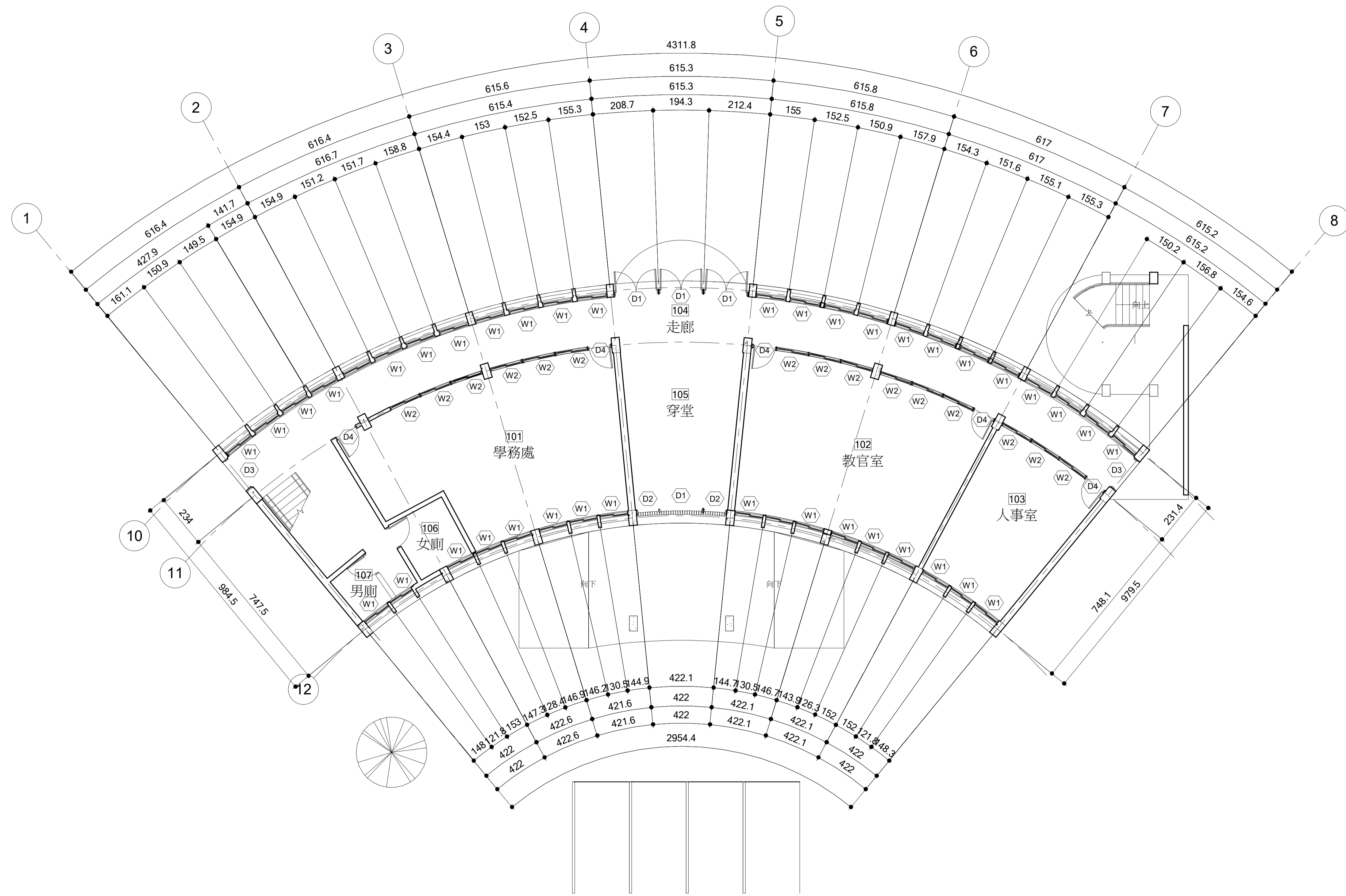
1 A-03 一樓平面圖 S= 1 : 100
