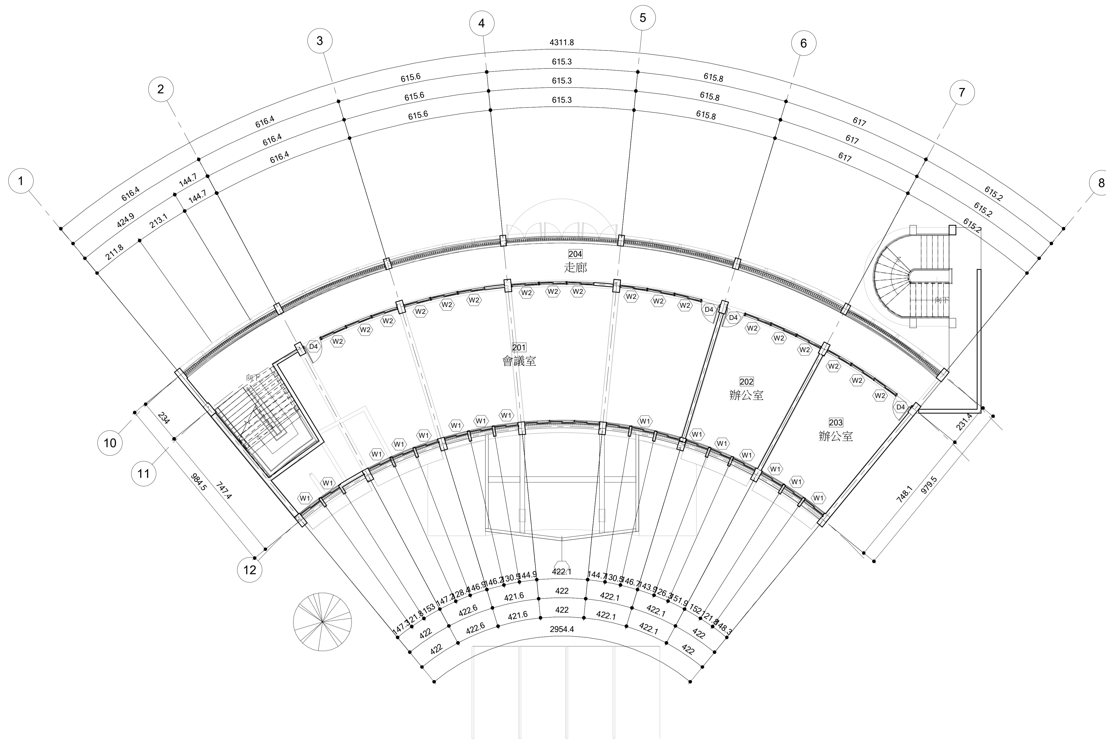
1 A-04 二樓平面圖 S= 1 : 100
