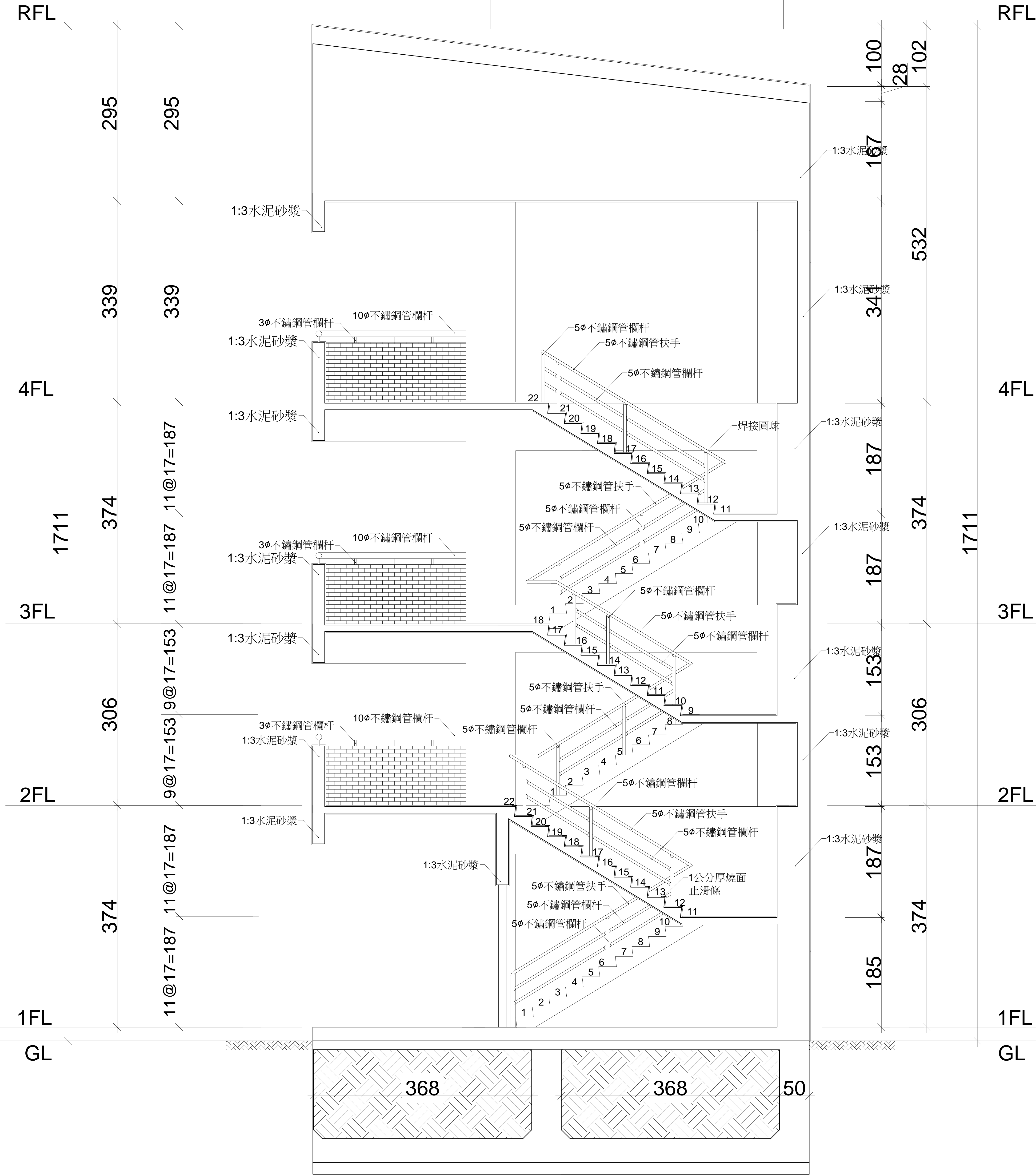
1 A-18 外掛樓梯剖面詳圖 S=1:30
