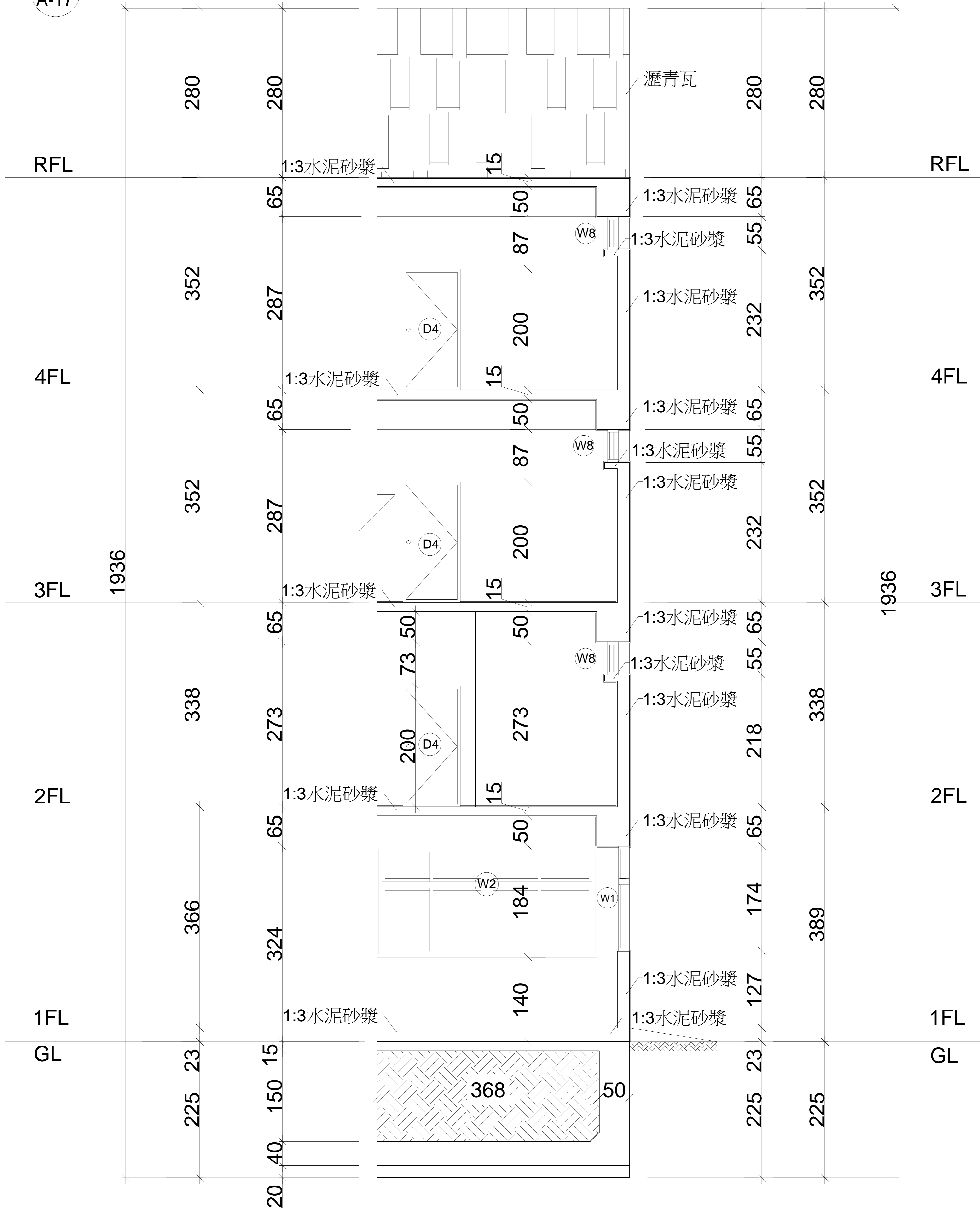
1 A-17 外牆剖面詳圖 S=1:30
